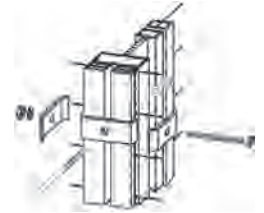
Pfosten-T-Anschluss mit T-Pfosten
