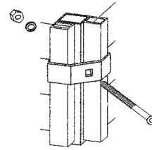
Pfosten-Eckanschluss mit Quadrat-Pfosten
